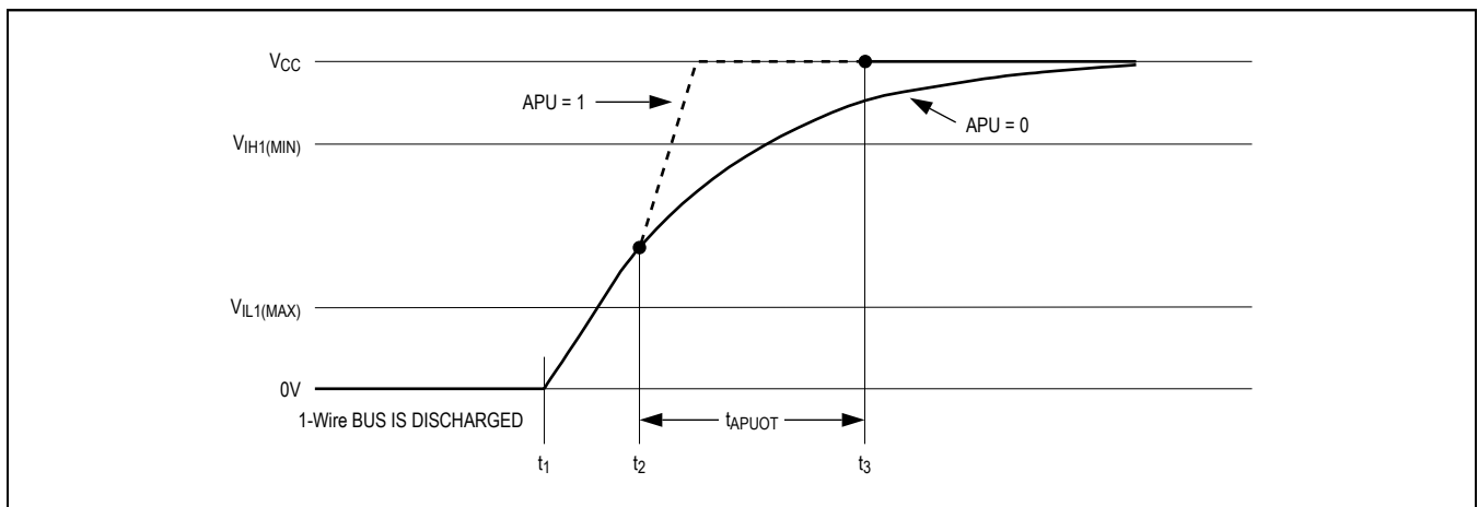
Figure 2. Rising Edge Pullup
